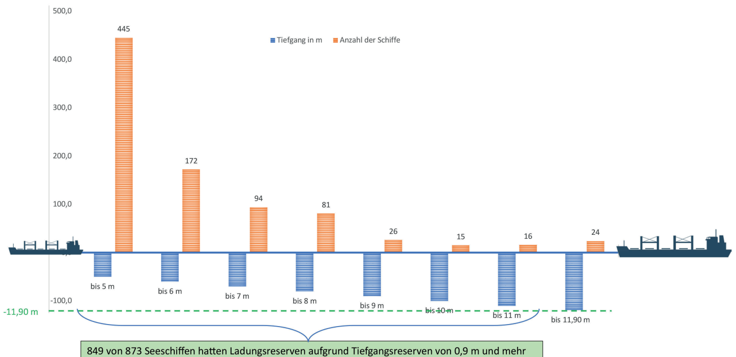
Abb. 2: Tiefgang der Brake anlaufenden Seeschiffe vom 01.01.2023 bis 31.12.2023 Daten aus fleetmon.com
