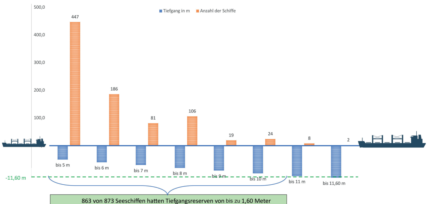
Abb. 1: Tiefgang der aus Brake auslaufenden Seeschiffe vom 01.01.2023 bis 31.12.2023 Daten aus fleetmon.com
